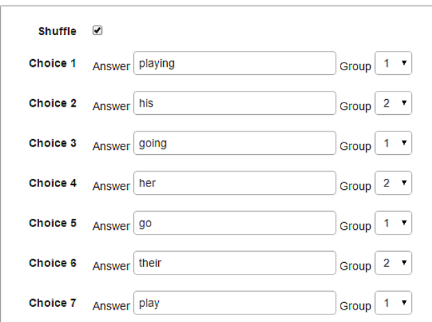
Fig. 4 Choice grouping
